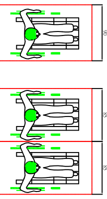
圖 703.1 Scale: 1:50 倍(5mm)
