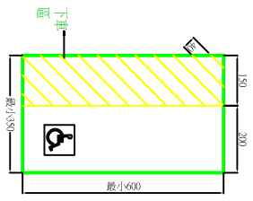
圖 804.1 Scale: 1:100 倍(5mm)
